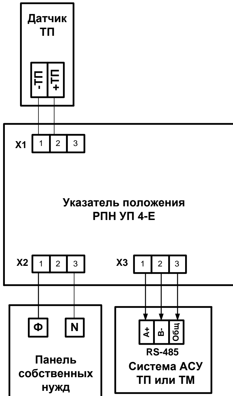
Рис. 4.1 Схема привязки УП 4-Е к приводу типа MR.
