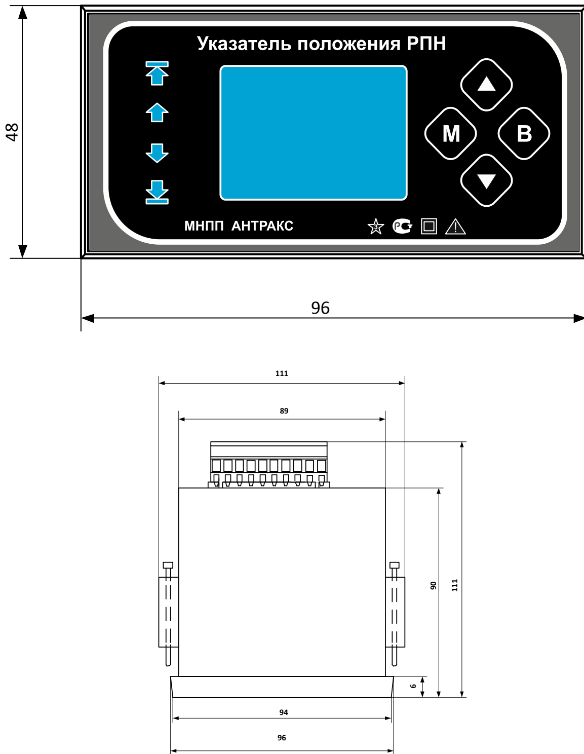
Рис. 1.1 Габаритные размеры щитового варианта указателя положения РПН УП 4-Е
